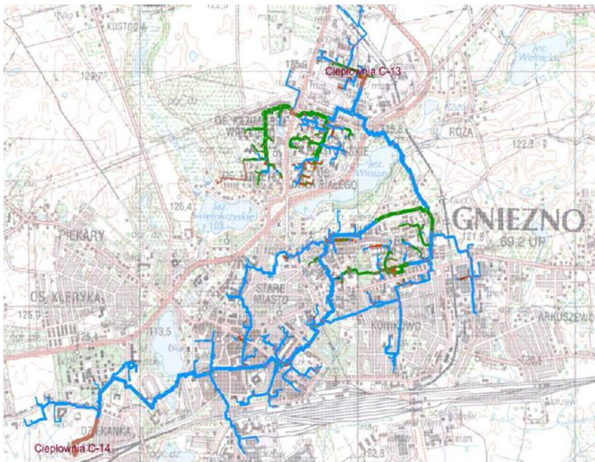
Rysunek 3 Schemat sieci ciepłowniczej
