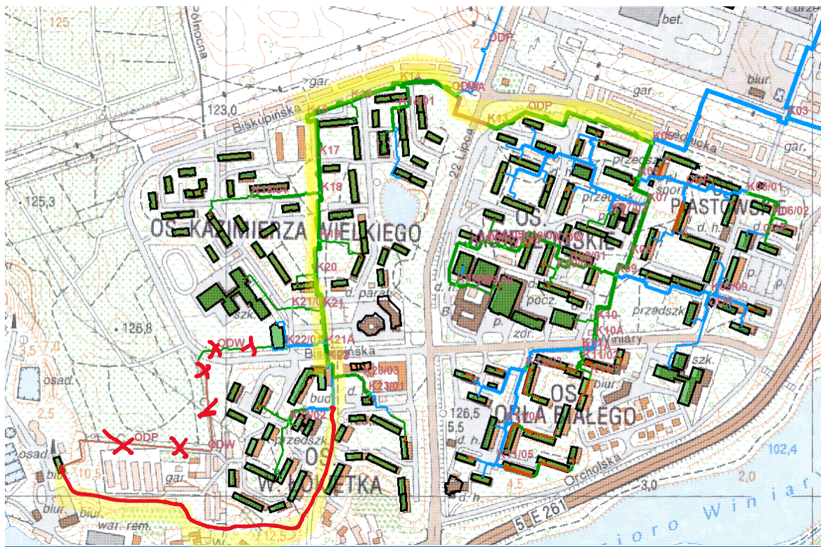
Rysunek 12. Odcinek sieci przeznaczony do modernizacji w związku z wyprowadzeniem mocy z nowego źródła.
