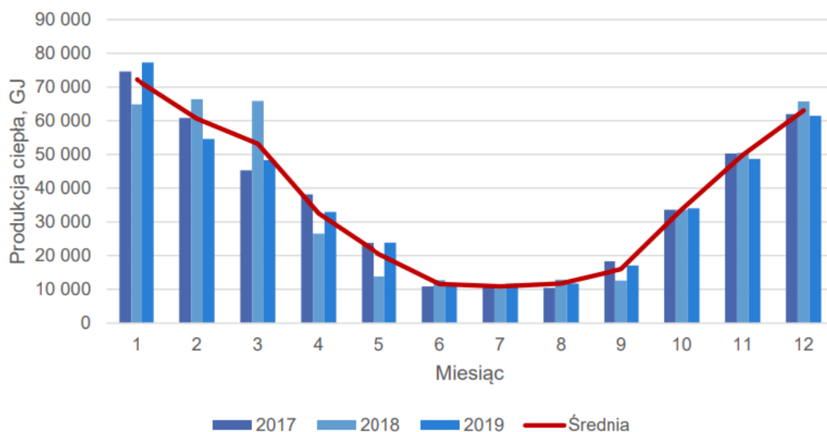
Rysunek 5. Produkcja ciepła przez ciepłownię C13 i C-14 w latach 2017-2019 (Project Energy)
