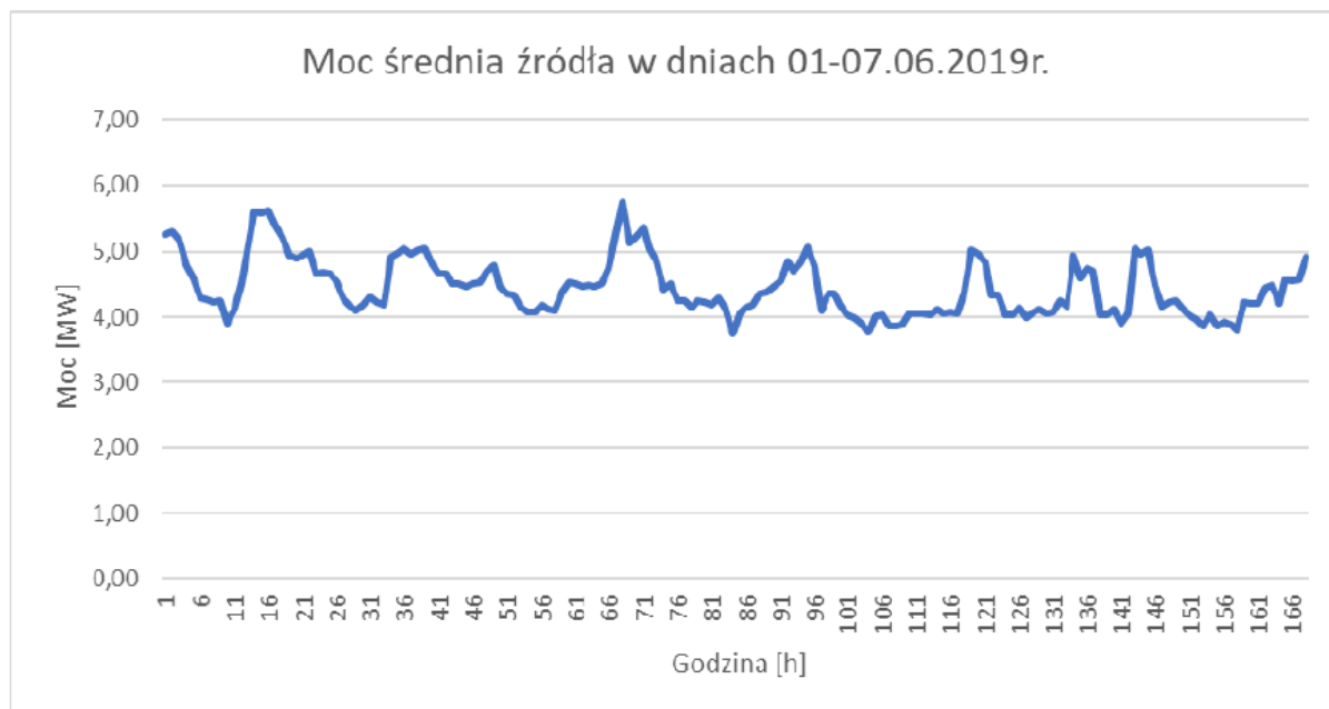
Rysunek 7. Moc średnia źródła w dniach 01-07.06.2019 ( opracowanie Derago)
